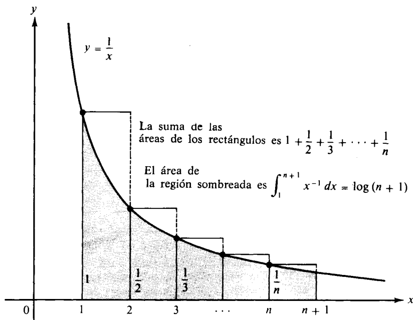
FIGURA 10.2 Significado geométrico de la desigualdad 1 + 1/2 + \cdots + 1/n \geq \log(n+1) .
